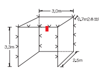
GF-445S 標準仕様
