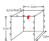
GF-325S 標準仕様
